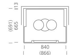
• METTE 1 Altezza 1015 mm Peso 1185 kg
