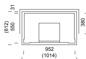
• JOYA-1 Altezza 1536 mm Peso 1610 kg
