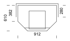
• RAIA SOLO-2 Altezza 1824 mm Peso 1635 kg
