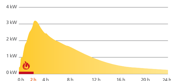
Rilascio del calore tipico delle stufe a iniettore ad accumulo termico
