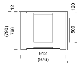
• MAMO SOLO 180-1 Altezza 1824 mm Peso 2290 kg
