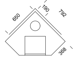
• JOYA ANGOLO Altezza 1536 mm Peso 1580 kg
