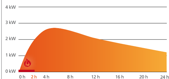
Rilascio del calore tipico delle stufe in pietra ollare ad accumulo termico
