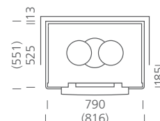
• ESSI 1 Altezza 1015 mm Peso 930 kg
