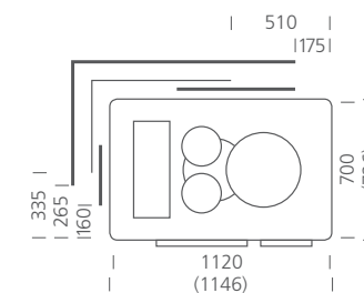
• EVA 1 Altezza 1015 mm Peso 1690 kg
