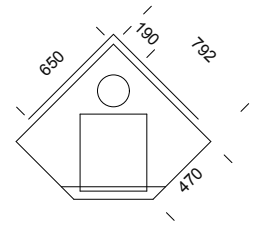
• RAIA ANGOLO SOLO Altezza 1824 mm Peso 1560 kg
