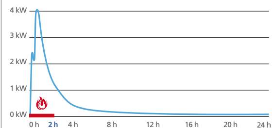
Rilascio del calore tipico delle stufe camino
